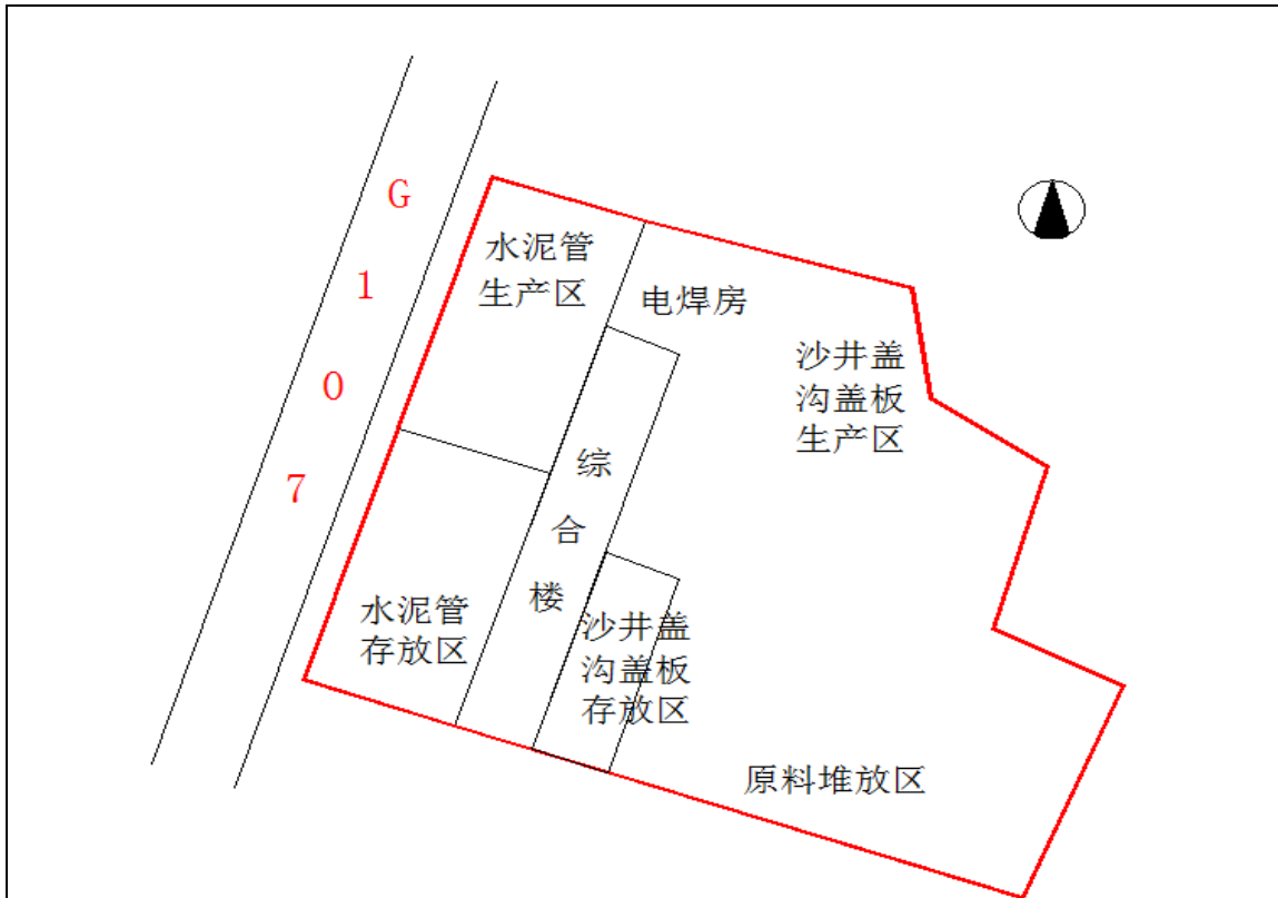
图3 项目总平面布置图
