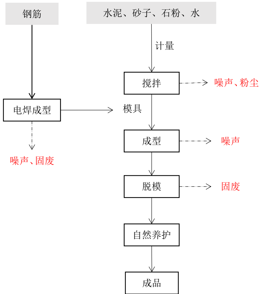
图 6 水泥管、沙井盖、沟盖板生产工艺流程及产污节点图
