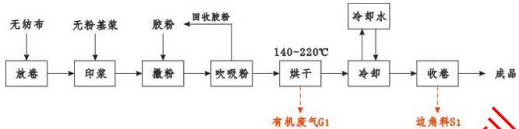
图 2-2 生产工艺流程及产污环节图
